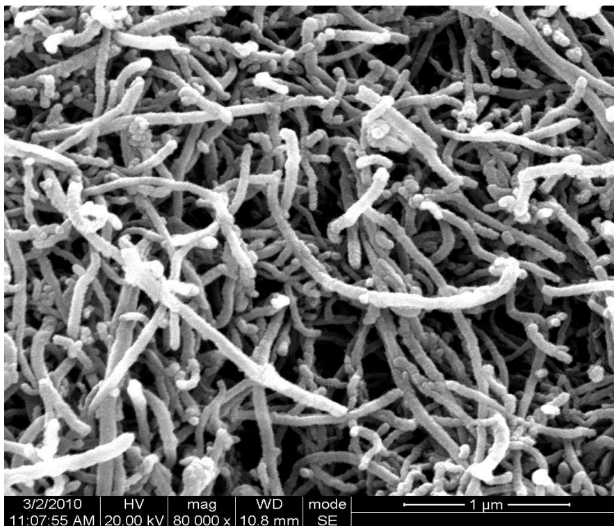
SEM
